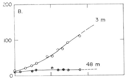
Fig. 2 — Distribuições de tamanho de partícula de sedimento em suspensão coletado por diferentes métodos de amostragem no rio Amazonas. Os números em cada curva são distâncias de amostras de 1 m abaixo da superfície. A) Amostras coletadas por coletor de profundidade integrada por profundidade total do rio (da superfície até ao leito e de volta à superfície) e pelo coletor integrado em uma única profundidade de 1 m abaixo da superfície (31 m acima do leito do rio). Cada curva representa uma combinação de duas amostras coletadas na parte central esquerda do canal, em São Paulo de Olivença, 22 de maio de 1977. B) Amostras coletadas por garrafas de Niskin de 30 L 3 m acima do leito do rio e na superfície do rio (48 m acima do leito do rio) no centro do canal próximo a Manacapuru, 22 de junho de 1976. C) Amostras coletadas por coletor point a 2 m, 24 m, 41 m e 54 m acima do leito do rio na parte central esquerda do canal em Óbidos, 14 de junho de 1976. Distribuições dos tamanhos de partícula a 41 m e 54 m não foram suficientes para garantir linhas separadas através de seus pontos. Amostra no local mais alto (54 m acima do leito) foi obtida na profundidade de 9 m abaixo da superfície da água.
