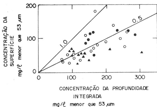
Fig. 1 — Relações entre concentrações de sedimento de grão fino em suspensão na superfície do rio e em amostras de profundidade integrada na calha do rio Amazonas perto de Iquitos, em São Paulo de Olivença, em Santo Antonio do Içá, em Itapeúba (perto de Coari), perto de Manacapuru, e em Óbidos. Amostras coletadas entre 20 de maio e 2 de junho de 1977. Os pontos estão codificados por profundidade do rio: círculos escuros, profundidades \leq 24 m; círculos abertos, 24-49m; triângulos, \geq 50 m. As linhas do gráfico não são de regressão, mas são linhas de referência para mostrar proporções de concentrações de superfície para profundidade integrada.
